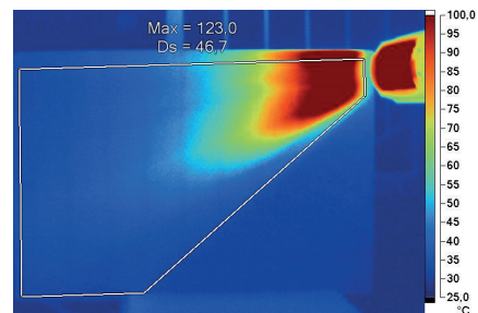
Toplotna slikanje brez varnostne razdalje ( min 20cm ) na stransko steno. Najvišja temperatura: 123,0 °C
