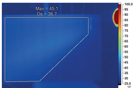
Termična slika na razdalji 50 cm. Maksimalna Temperatura: 45,1 °C
