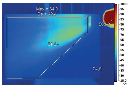
Termična slika na razdalji 20 cm. Maksimalna Temperatura: 64,0 °C
